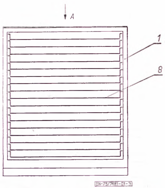
Rys. 3. Regal z deskami (wskaźniki liczbowe wg tabeli)
