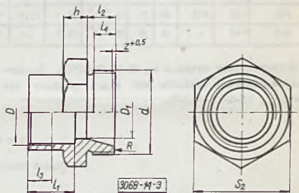
Rys. 3. Korpusy redukcyjne typu KWr i KPr toczone
