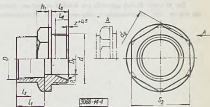
Rys. 4. Korpusy redukcyjne typu KWr i KPr odlewane i prasowane
