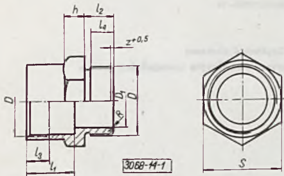
Rys. 1. Korpusy typu KW i KP toczone
