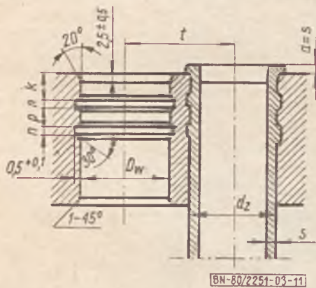
Rys. 11. Sposób mocowania R5
