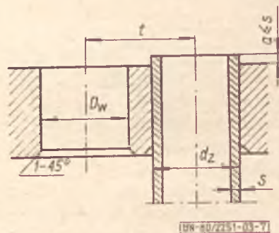
Rys. 7. Sposób mocowania R1
