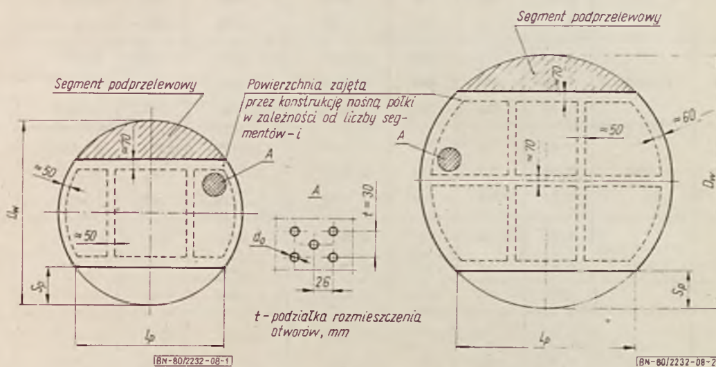
Rys. 1. Półka sitowa jednoprzelawowa z dużymi otworami dla D_w = 600 \div 2600 mm
