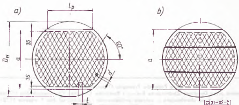
Rys. 2. Półki sitowe jednoprzelawowe: a) półka niedzielona dla średnic 600 i 800 mm, b) półka dzielona dla średnic od 1000 do 4000 mm
