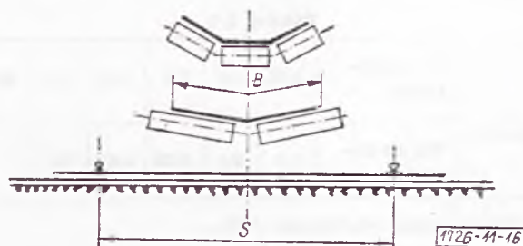
Rys. 16. Rozstaw osi szyn członów przesuwnych
