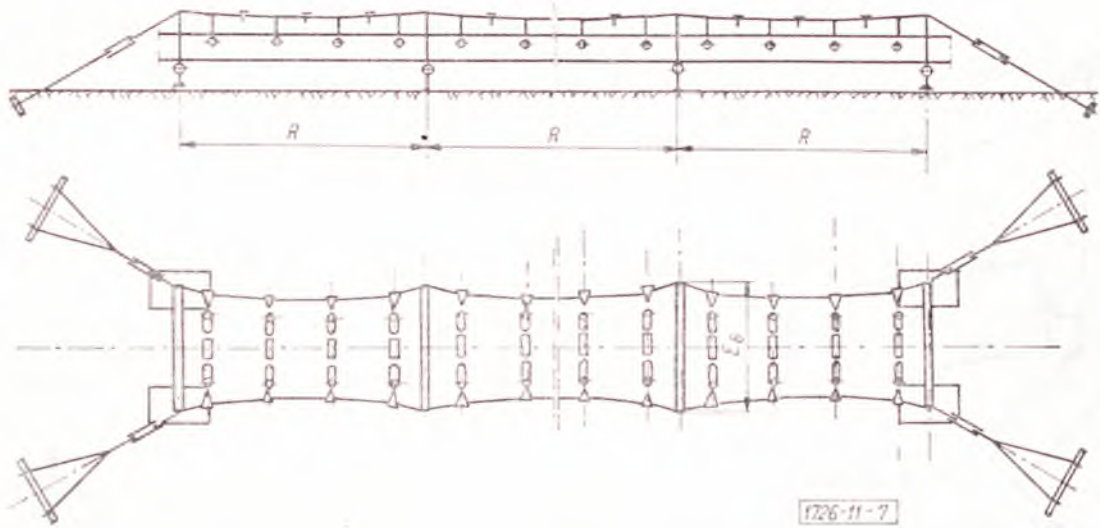
Rys. 7. Człon linowy
