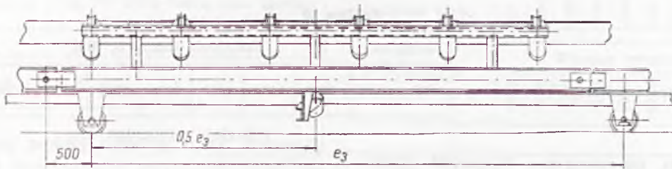
Rys. 10. Człon sztywny przejezdny
