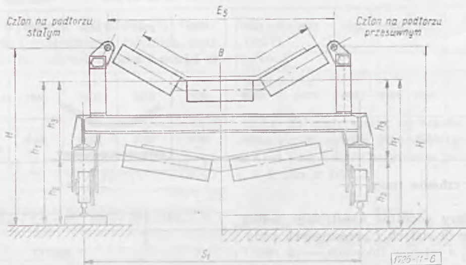
Rys. 6. Człon przejezdny. Konstrukcja przykładowa
