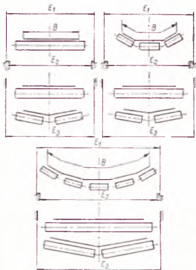
Rys. 1. Wymiary poprzeczne konstrukcji nośnej członów z zestawami sztywnymi
