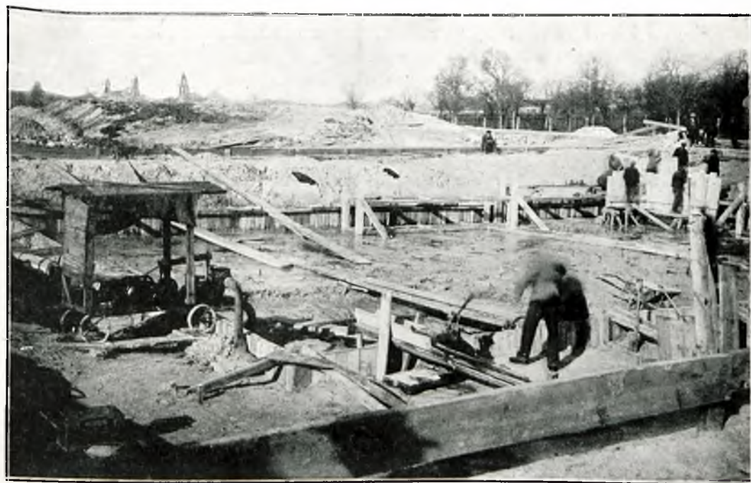
Fot. 2. Piotrków. Kanalizacja. „Oczyszczalnia ścieków” — fundamentowanie zbiornika „Imhoffa” (str. 192)
