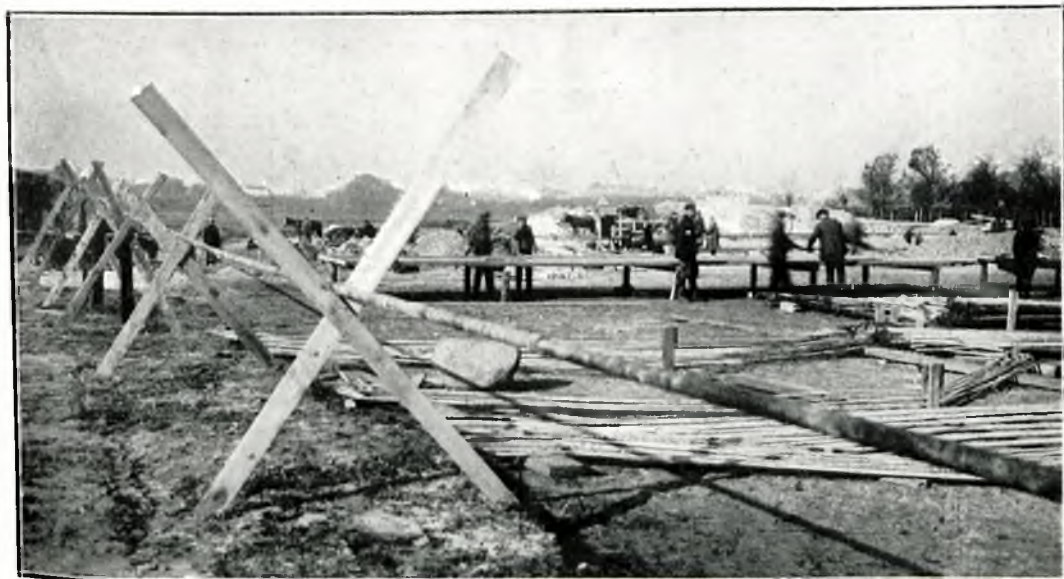
Fot. 1. Piotrków. Kanalizacja. Oczyszczalnia ścieków w budowie—widok ogólny (str. 192).
