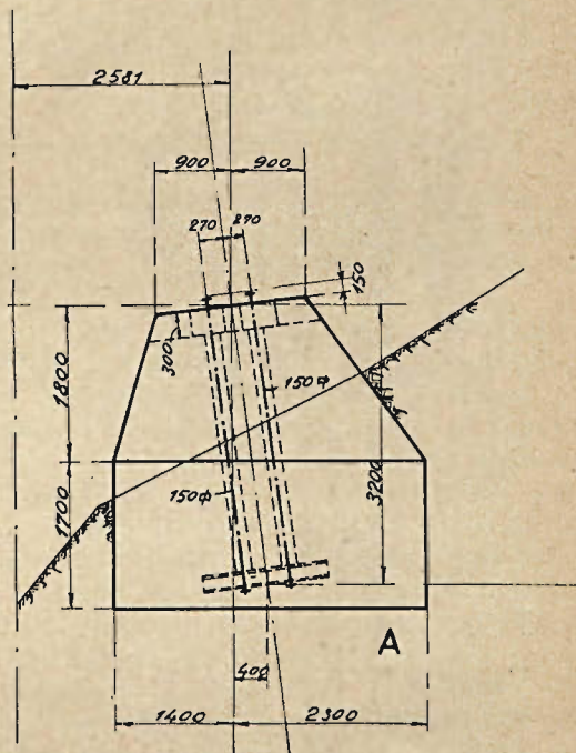
Rys. 14. Fundament A wieży podporowej N 6.
