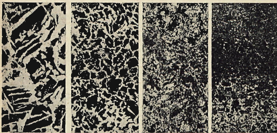
Rys. 5 a-d. a) Struktura szyny 255° Br. b) Szyna po ulepszeniu zapomocą palnika tleno-acetylenowego. c) Przejście od szyny do warstwy nałożonej w stanie surowym 179° Br. d) To samo po ulepszeniu 205° Br.
