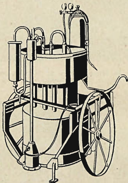
Rys. 6. Wytownica acetylenowa.
