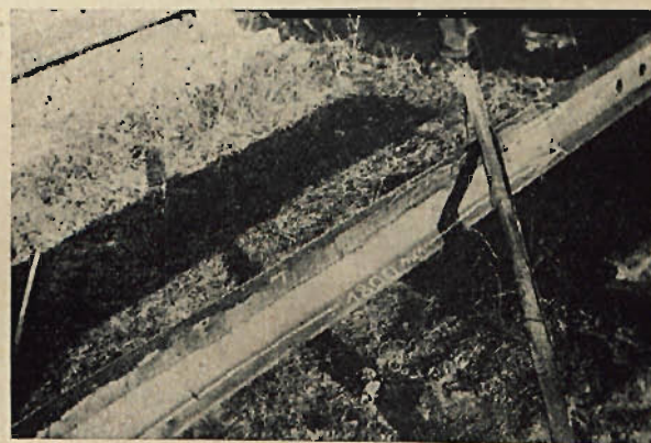
Rys. 4. Po 10-ciu uderzeniach młotem szyna, uwidoczniiona na rys. 3, rozłupała się. Część odłupaną widać umieszczoną obok.
