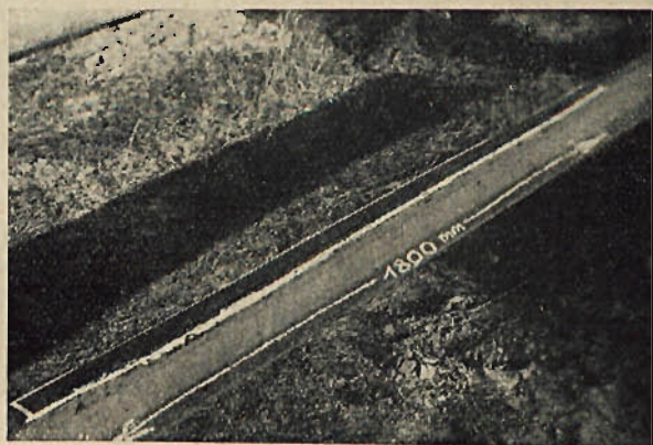
Rys. 3. Na długości 1,8 m szyna miała podłużne pęknięcie, sięgające włąb aż do szyjki.
