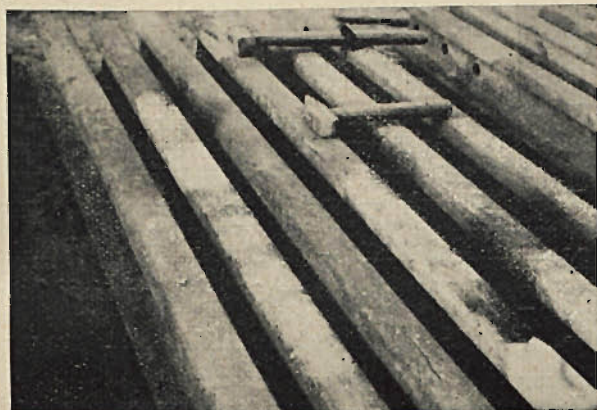
Rys. 21. Szyny po napawaniu. Widać jaśniejsze miejsca napawania raków.
