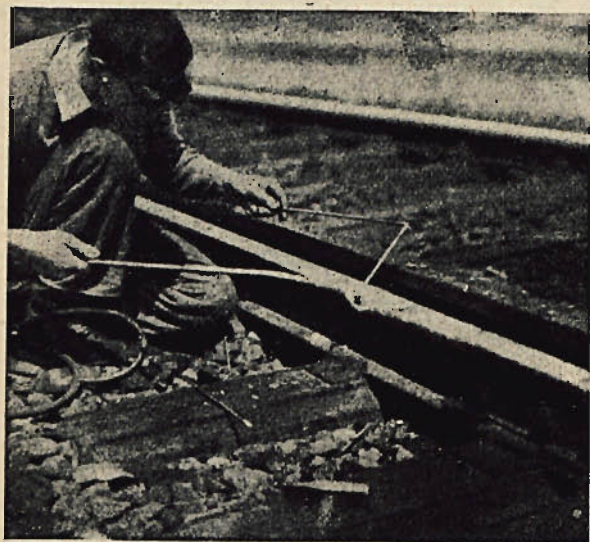
Rys. 18. Napawacz przy pracy napawania.
