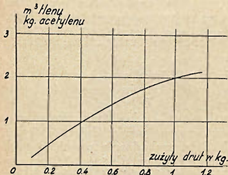
Rys. 22. Zużycie gazu w zależności od ilości nałożonego metalu.
