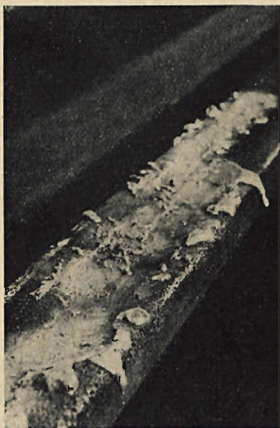
Rys. 13. Szyna po wypaleniu raka.
