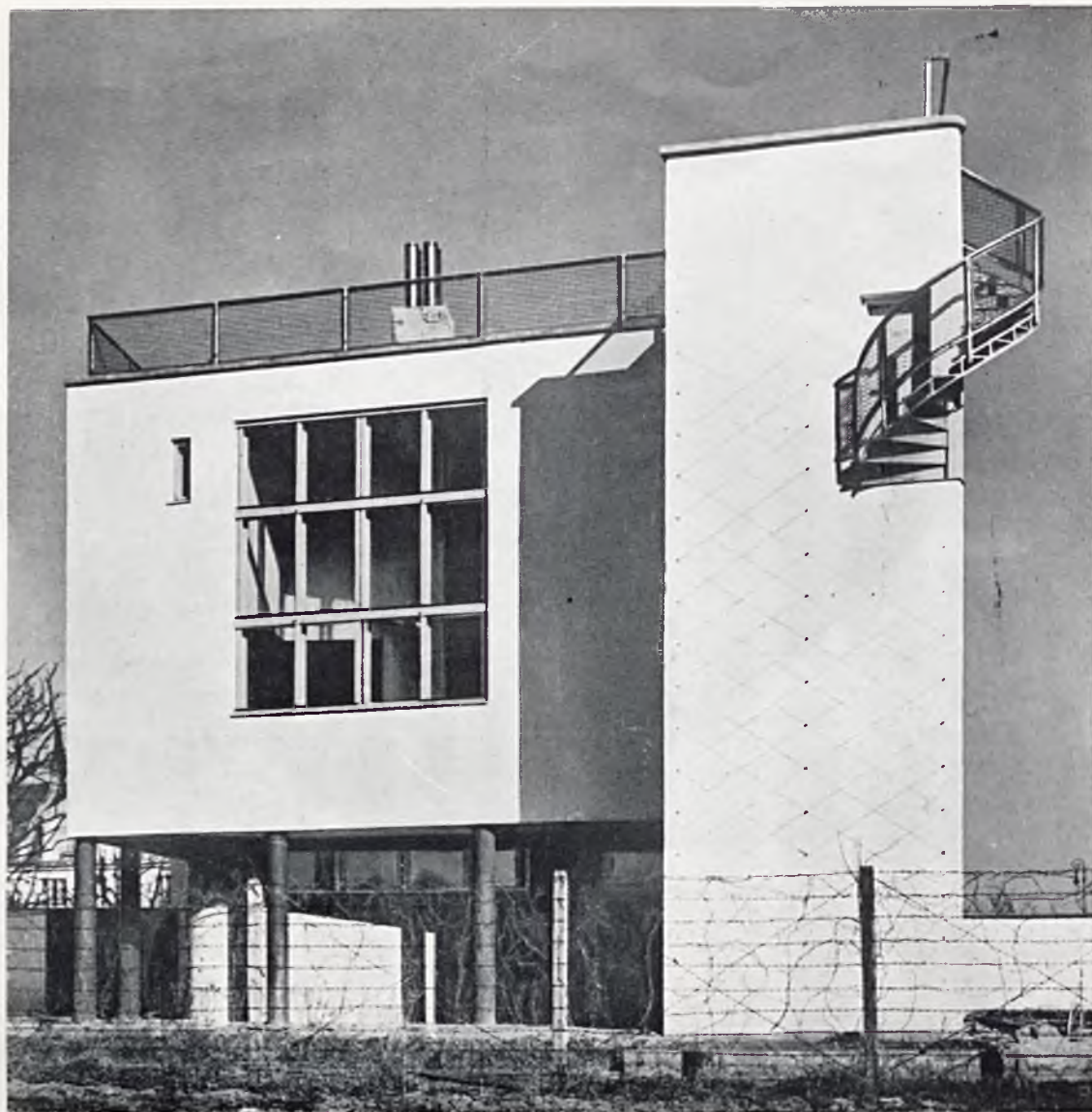
ARCH. BOHDAN LACHERT (SARP), ARCH. JÓZEF SZANAJCA (SARP) Dom jednorodzinny. Maison pour une famille. One-family House. Einfamilienhaus. Casa per una famiglia. Warszawa
