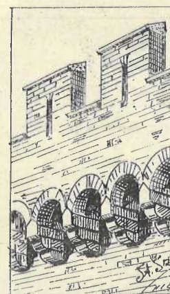
Rys. 64. Hurdyca na murach zamków średniowiecznych Zachodu, jako dalsze rozwinięcie zasady nawieszania ścian (por. z rys. 60, 61, 62).
