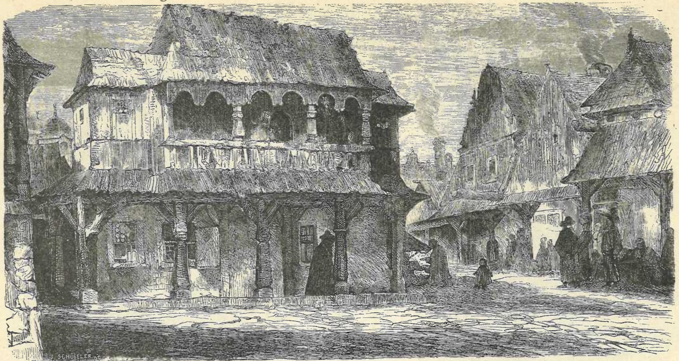
Rys. 17. Domy podcieniowe na rynku w Wiśniczu przed pożarem w 1863 r. (Rys. J. Matejki, Tyg. Illustr. 1871). Daszki okapowe na podcieniach i przy szczytach, szczyty cofnięte od lica ścian, dachy łamane o jednakowej pochyłości nadają tym budowlom wybitny typ polski.
