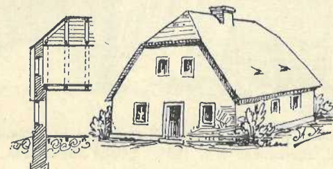
Rys. 26. Dom murowany z dachem naczółkowym, t. zw. „pruskim.“ Ściana szczytowa bez zewnętrznej odsadzki, a więc i bez okapu-daszku przyźbowego. Ściana poddasza i przyziemia tworzą jedną płaszczyznę pionową (patrz przekrój).
