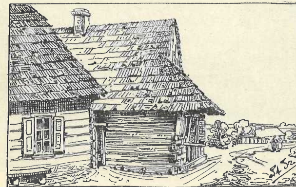
Rys. 55. Chata w Inowłodziu nad Pilicą, pow. Rawski. Trójkąt szczytowy silnie od lica ściany cofnięty.
