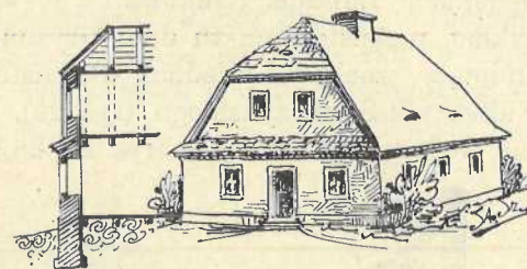
Rys. 25. Dom murowany z dachem naczółkowym polskim. Zewnętrzna odsadzka ściany szczytowej pokryta okapem-daszkiem przyźbowym. Ściana poddasza cofnięta od pionu lica ściany przyziemia (patrz przekrój).
