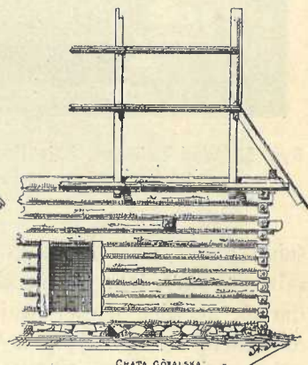
Rys. 8. Chata góralska. Widok boczny.
