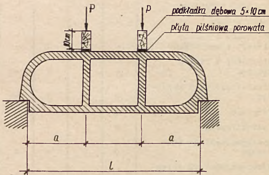
Rys. 3. Przykładowe obciążenie dwiema siłami skupionymi
