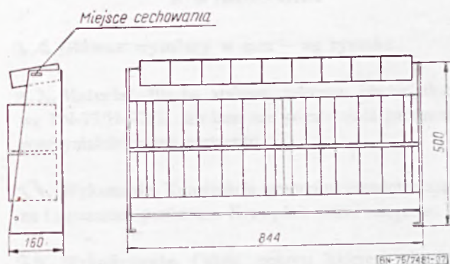
Nadbudówka do przechowywania justunku
