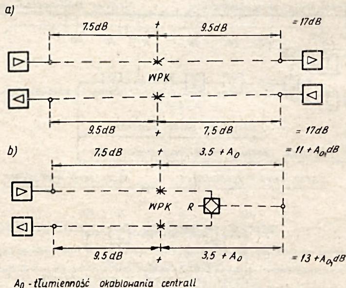
Rys. I-6. Tłumienności odcinka stacyjnego centrali międzynarodowej przy 800 Hz: a) przy połączeniu łączy dwutorowych, b) przy połączeniu łączy dwutorowego z łączem jednorowym
