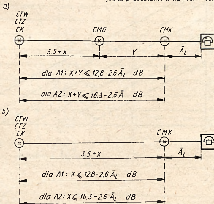
Rys. I-16. Zestaw łączy od centrali międzymiastowej do aparatu telefonicznego: a) w przypadku połączenia CMK z centralą międzymiastową poprzez CMG, b) w przypadku bezpośredniego połączenia CMK z centralą międzymiastową
