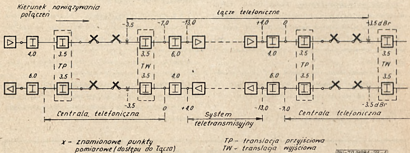
Rys. 1. Przykład struktury łącza telefonicznego
