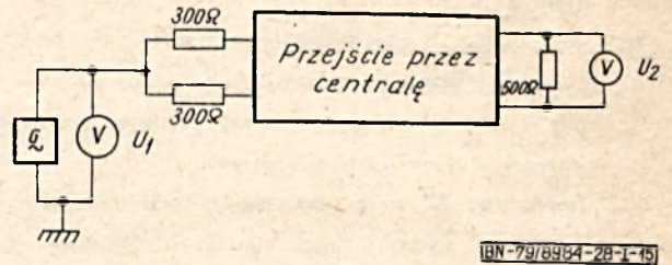
Rys. I-15. Układ do pomiaru asymetrii przejścia
