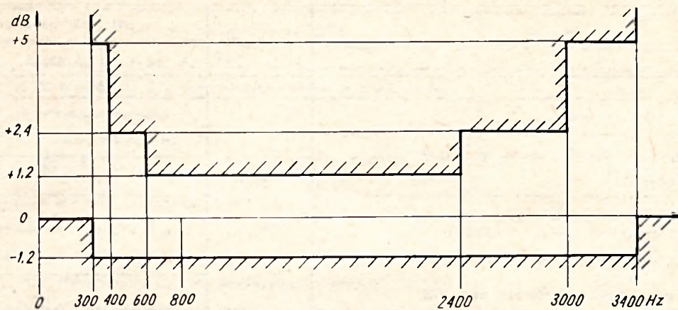
Rys. 4. Dopuszczalne zniekształcenia tłumieniowe łącza międzymiastowego przy ruchu bezpośrednim
