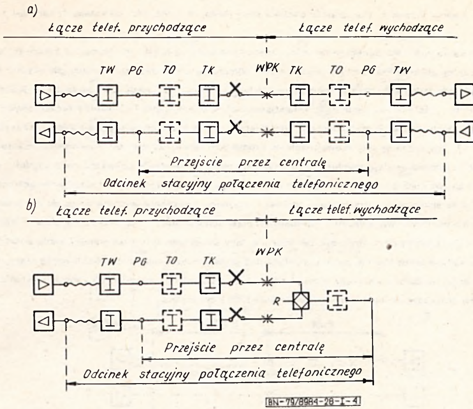
Rys. 1-4. Odcinki stacyjne połączenia telefonicznego przy dwutorowej komutacji łączy w centrali telefonicznej: a) połączenie dwóch łączy dwutorowych, b) połączenie łączy dwutorowego z jednotorowym
