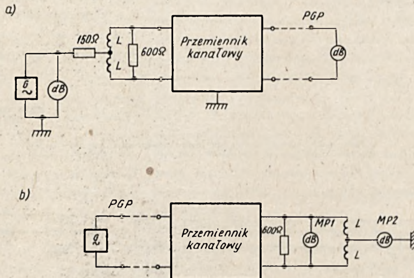
Rys. 1-14. Układy pomiarowe asymetrii względem ziemi: a) wejście kanału, b) wyjście kanału
