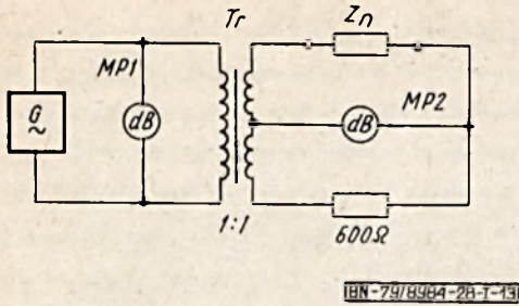
Rys. 1-13. Układ do pomiaru tłumienności niedopasowania
