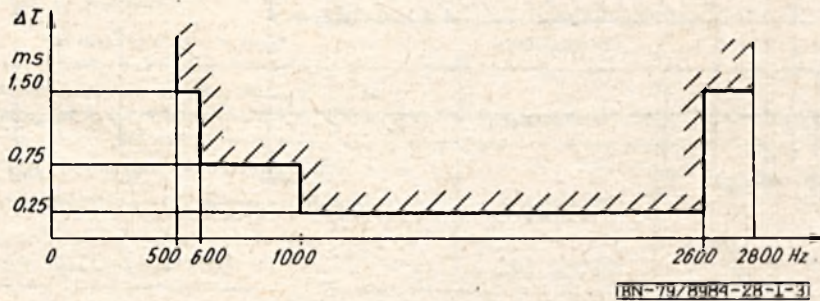
Rys. 1-3. Zniekształcenia opóźnieniowe kanału cyfrowego w odniesieniu do najmniejszej wartości opóźnienia w przesyłanym paśmie
