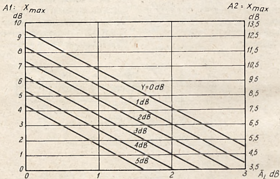
Rys. I-17. Diagram do wyznaczania tłumienności łącza pośredniczących (zgłoszeniowo-połączeniowych) i międzycentralowych
