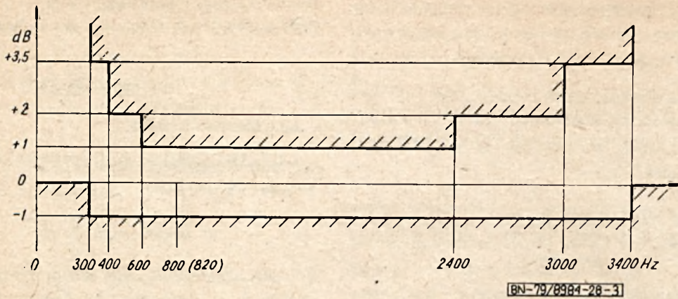
Rys. 3. Dopuszczalne zniekształcenia tłumieniowe łącza międzynarodowego lub międzymiastowego tranzytowego
