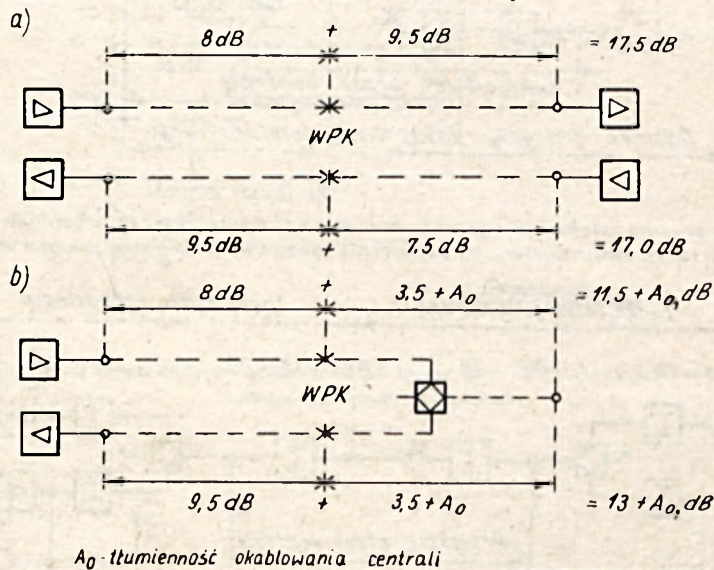
Rys. I-6. Tłumienności odcinka stacyjnego centrali międzynarodowej przy 800 Hz: a) przy połączeniu łączy dwutorowych, b) przy połączeniu łączy dwutorowego z łączem jednorowym
