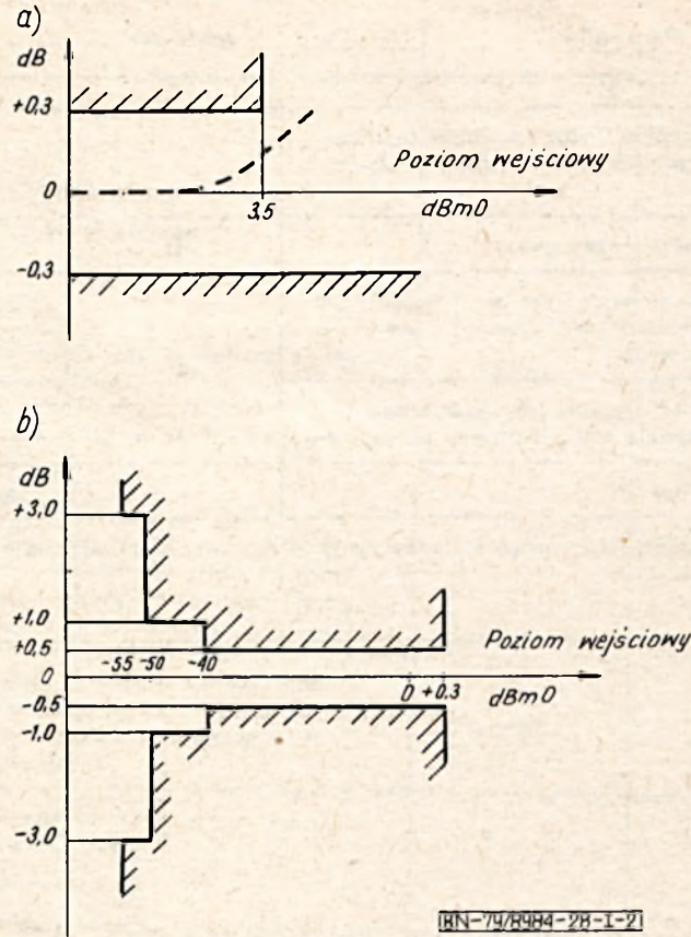
Rys. 1-2. Charakterystyka amplitudowa przy połączeniu na siebie urządzeń nadawczych i odbiorczych: a) kanału analogowego, b) kanału cyfrowego
