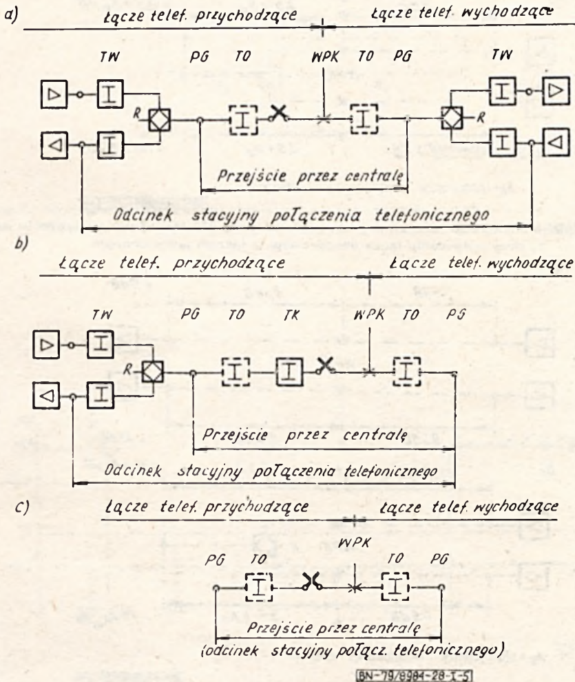
Rys. 1-5. Odcinki stacyjne połączenia telefonicznego przy jednotorowej komutacji łączy w centrali telefonicznej: a) połączenie dwóch łączy dwutorowych, b) połączenie łączy dwutorowego z jednotorowym, c) połączenie dwóch łączy jednotorowych
