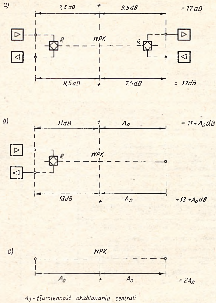
Rys. 1-8. Tłumienność odcinka stacyjnego centrali telefonicznej o komutacji jednorowej przy 800 Hz: a) przy połączeniu łączy dwutorowych, b) przy połączeniu łączy dwutorowego z jednorowym, c) przy połączeniu łączy jednorowych
