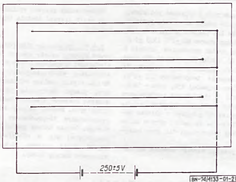
Rys. 2. Schemat obwodu elektrycznego do badań
