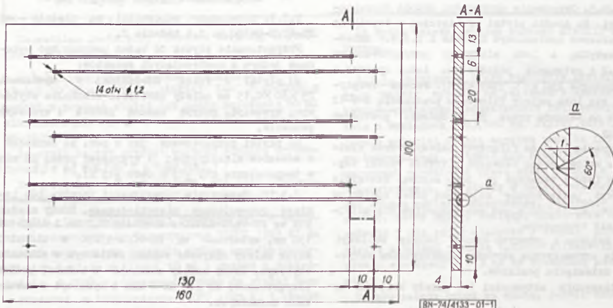
Rys. 1. Płytko do badań
