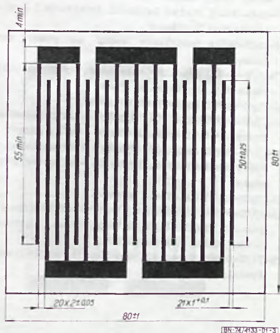
Rys. 3. Płytki do badań
